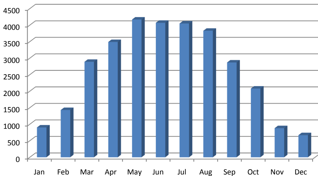
Генерація електроенергії сонячною станцією потужністю 30 кВт протягом року (енерговиробіток кВт*год. по місяцях)
